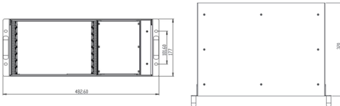
适用型号: B-542.3B, B-542.3C, B-543.3B, B-543.3C, B-544.3B, B-544.3C 尺寸单位:mm
